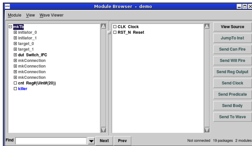
Figure 16: Module Browser
